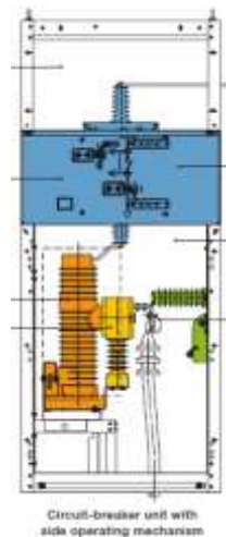
Figura 9. Celda de protección
