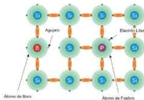
Figura 2. Estructura atómica células solares
