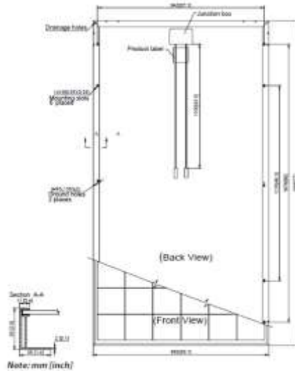
Figura 5. Vista posterior módulo fotovoltaico
