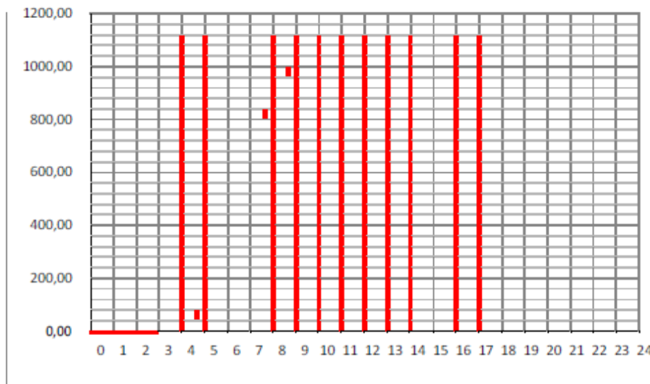
Figura 21. Curva de funcionamiento del transformador el 20 de Agosto
