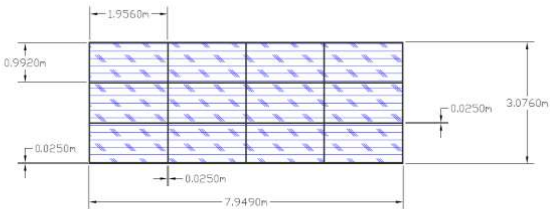
Figura 17. Disposición de los paneles sobre la estructura soporte
