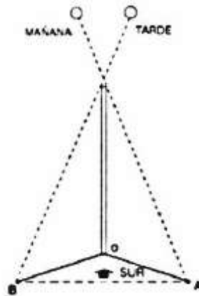
Figura 11. Localización del Sur geográfico
